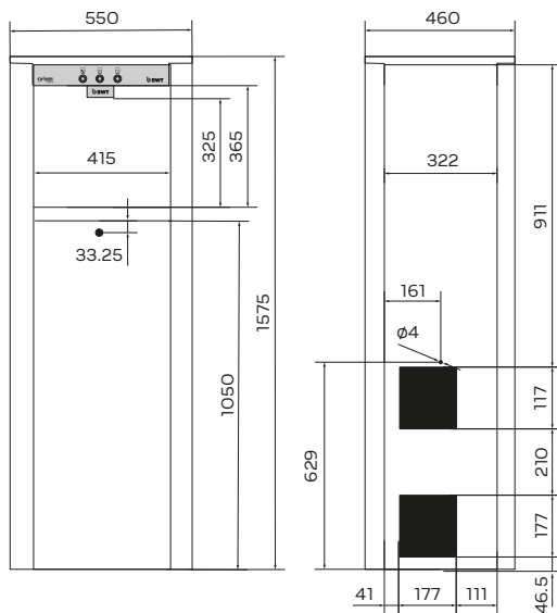
Ill. 4: Cotes et dimensions du BWT AQA drink Pro 3 en millimètres
