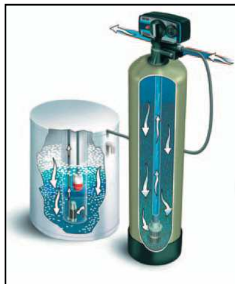
2. ábra – egyoszlopos készülék működési vázlat
